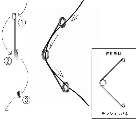
ワイヤ取付手順
