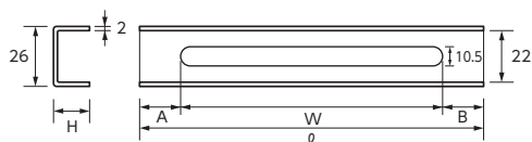
寸法図
