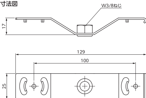
寸法図
