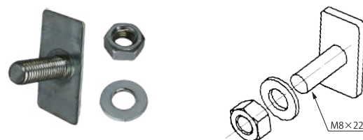
回転止めボルトセット
