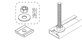
ND-1・2 取付例
