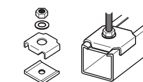
ND-1・2 取付例
